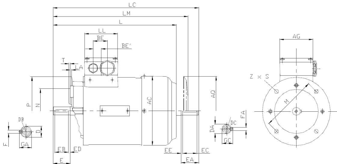
Fuß- Flanschbaufornen feet / flange type of construction
