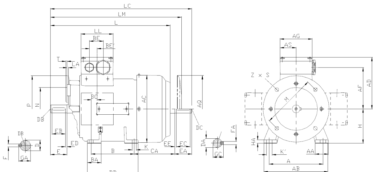
Fuß- Flanschbaufornen feet / flange type of construction
